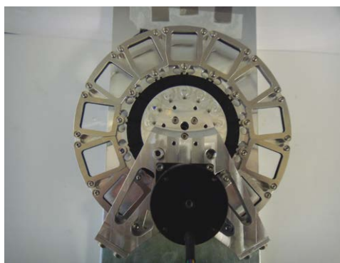
IM Janus Filter Wheel for JUICE ESA
